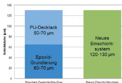
Graf 1 - Porovnává nový jednovrstvý systém s dosavadní standardní dvouvrstvou skladbou High Solid epoxidového základu a PU horního laku.
